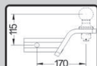
CÓDIGO PONTEIRA K982PR CÓDIGO 4666
