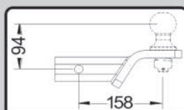
CÓDIGO PONTEIRA K978PR CÓDIGO 4665
