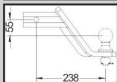
CÓDIGO PONTEIRA K982PR CÓDIGO 4666
