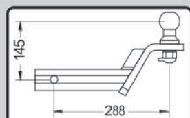
CÓDIGO PONTEIRA K983PR CÓDIGO 4664
