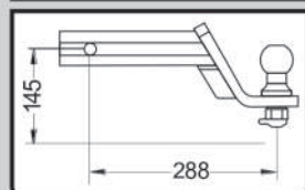
CÓDIGO PONTEIRA K981PR CÓDIGO 5162
